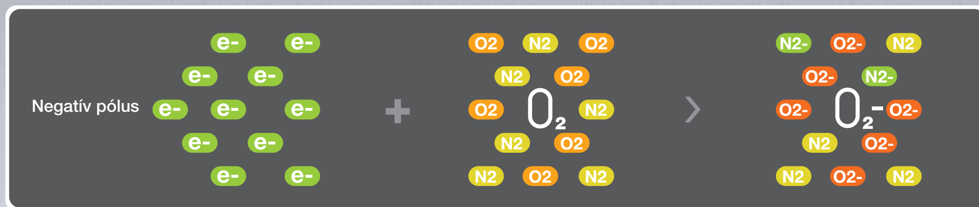
Elektron nyaláb a levegőben
